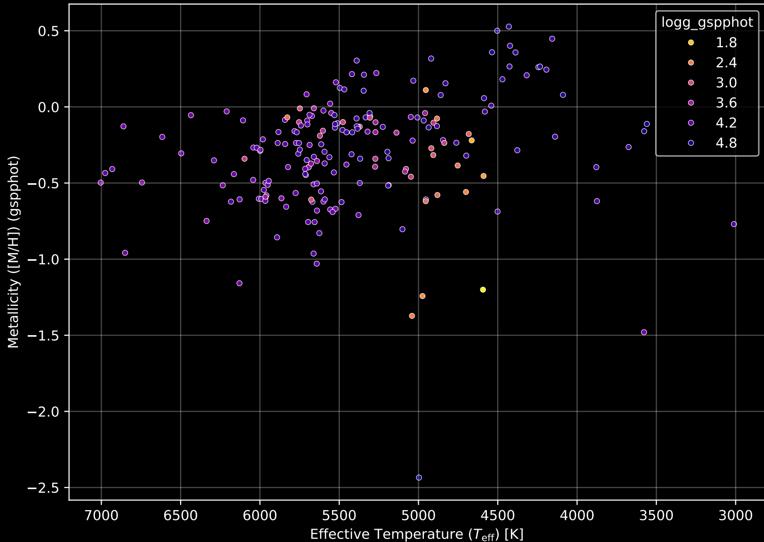
APOGEE DR17 Field: [335+61_btx] Stellar Population Parameters (n= 200)
